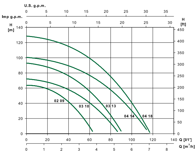
Curvas de funcionamiento a 2900 rpm
