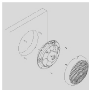
Montaje en pared: mediante cuatro tornillos que sujetan el cuerpo interior en la propia pared. Diámetro de perforación (mm) HCM-150 N: 183 a 188 HCM-180 N: 220 a 225 HCM-225 N: 262 a 267
