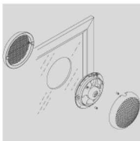
Montaje en cristal: mediante dos tornillos que sujetan el cuerpo interior con la brida de protección exterior. Espesor máximo (3 a 6 mm) Diámetro de perforación (mm) HCM-150 N: 183 a 188 HCM-180 N: 220 a 225 HCM-225 N: 262 a 267
